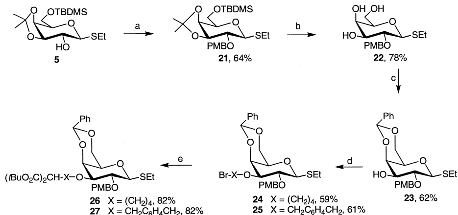
Scheme 2. (a) PMBCl, NaH, DMF; (b) AcOH, THF; (c) PhCH(OCH_3)_2 , PTSA, MeCN; (d) Br-X-Br , NaH, DMF; (e) NaCH(CO_2tBu)_2 , THF, DMF.
