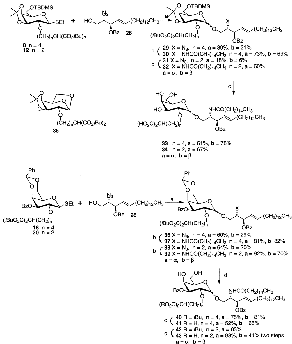
Scheme 3. (a) DMTST, 2,6-di- t Bu-4-Me-pyridine, solvent, mol. sieves; (b) (1) H 2 S, pyridine, H 2 O; (2) CH 3 (CH 2 ) 14 COCl, NaOAc, THF; (c) TFA 90%; (d) TFA 90%, CH 2 Cl 2 .
