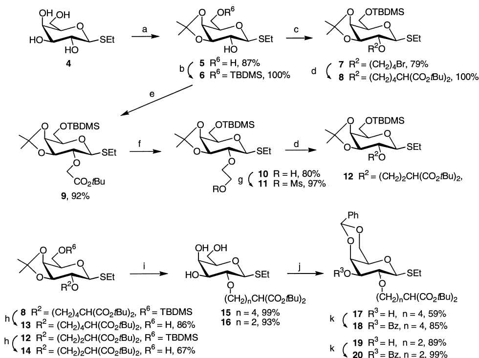
Scheme 1. (a) CH_3C(OCH_3)_2CH_3 , PTSA; (b) TBDMSCl, pyridine, DMAP; (c) NaH, Br(CH_2)_4Br , DMF; (d) NaCH(CO_2tBu)_2 , THF, DMF; (e) NaH, BrCH_2CO_2tBu , DMF; (f) LAH, THF; (g) MsCl, NEt_3 , CH_2Cl_2 ; (h) nBu_4NF , THF; (i) 3 N HCl, THF; (j) PhCH(OCH_3)_2 , MeCN, PTSA; (k) BzCl, py, DMAP.
